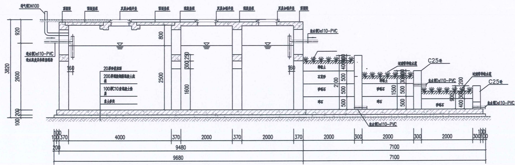
1-1 1:50
