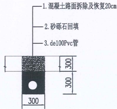
入户管管槽开挖及恢复 涉及入户管长1400m
