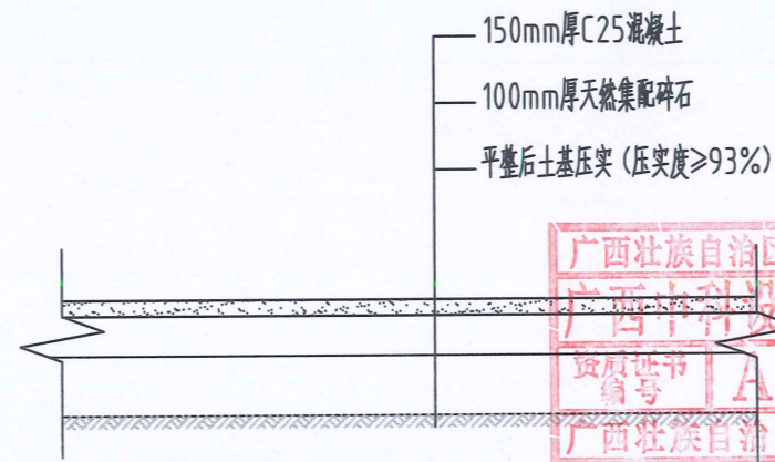
硬化地面恢复做法
