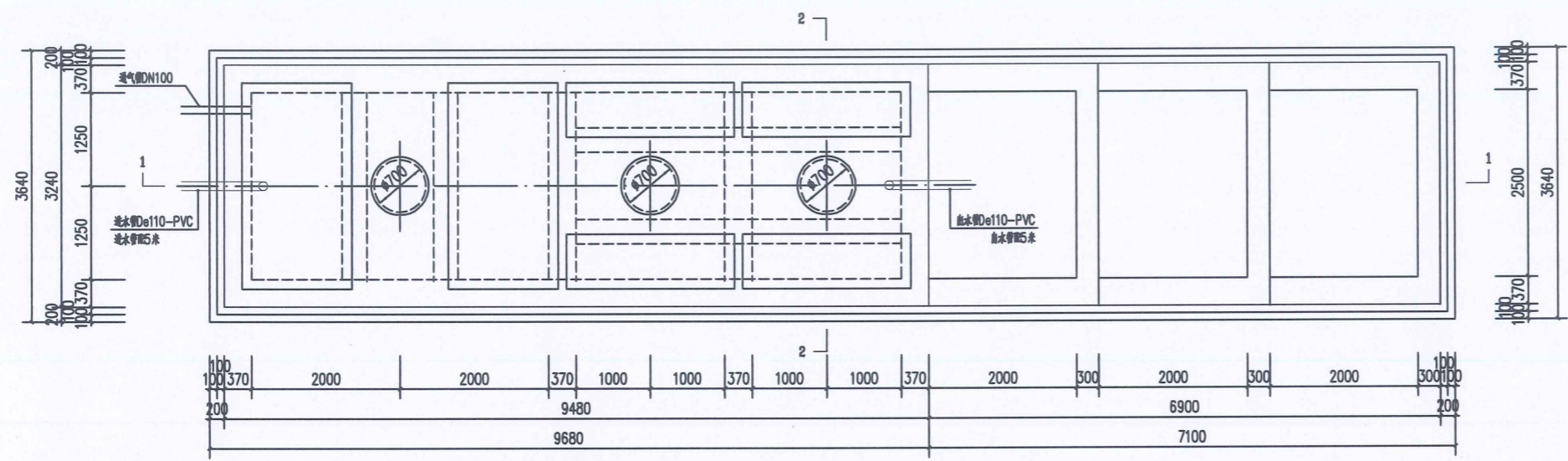
砖砌化粪池平面图 1:50
