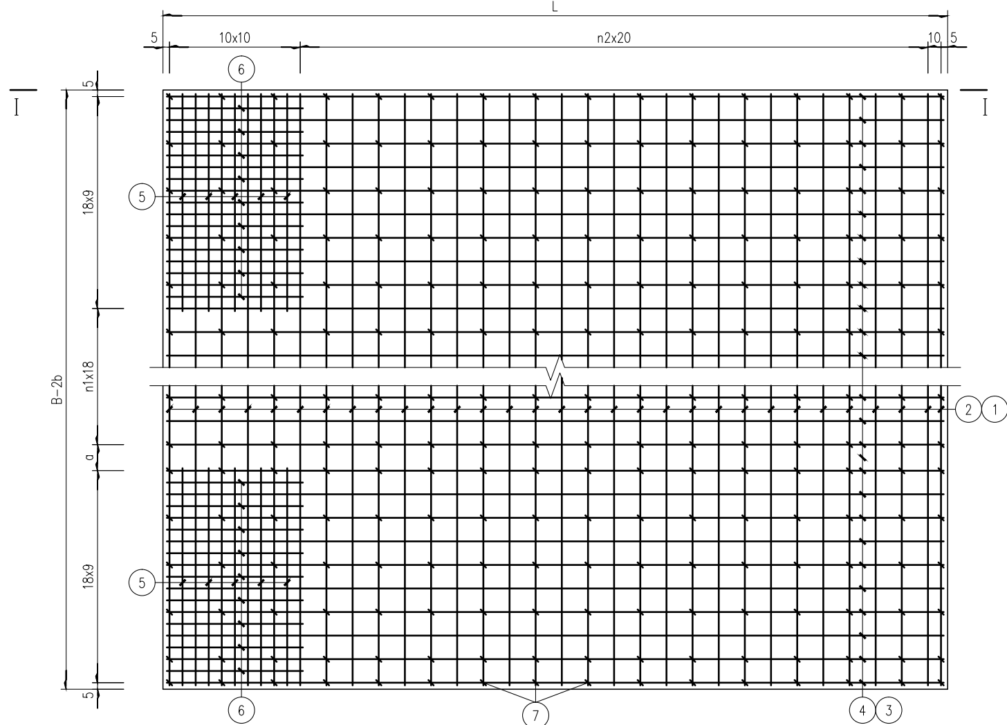
平面 1:40
