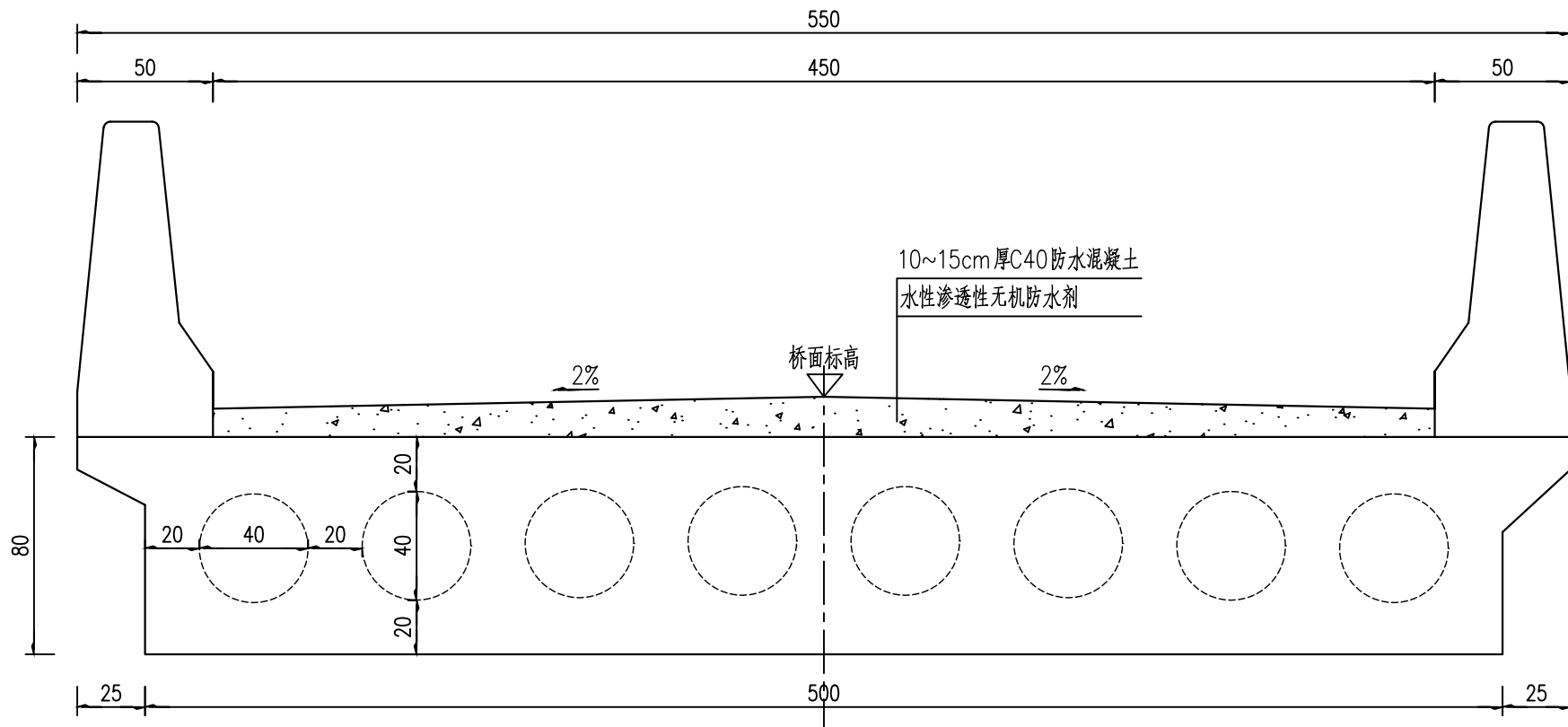
上构跨中断面图 1:25
