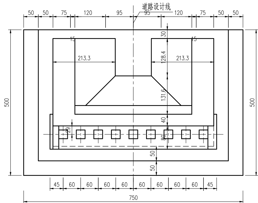
平面 1:75
