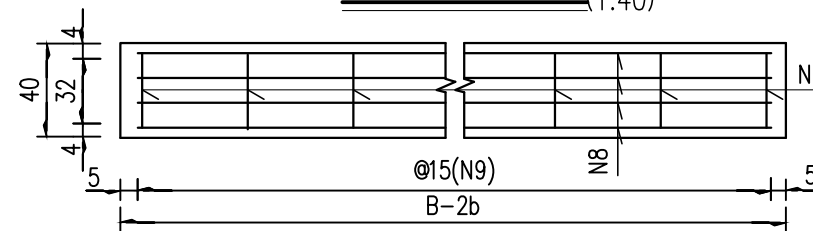
枕梁钢筋构造图 (1:40)
