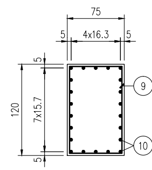
侧墙混凝土横断面 1:50
