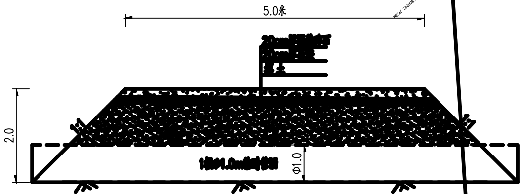
临时便道断面图(跨河)
