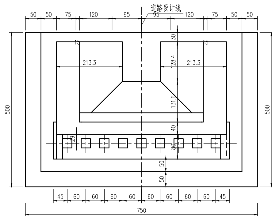
平面 1:75
