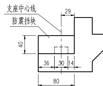
側面 1:50
