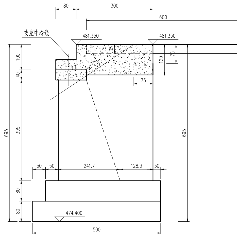
側面 1:75
