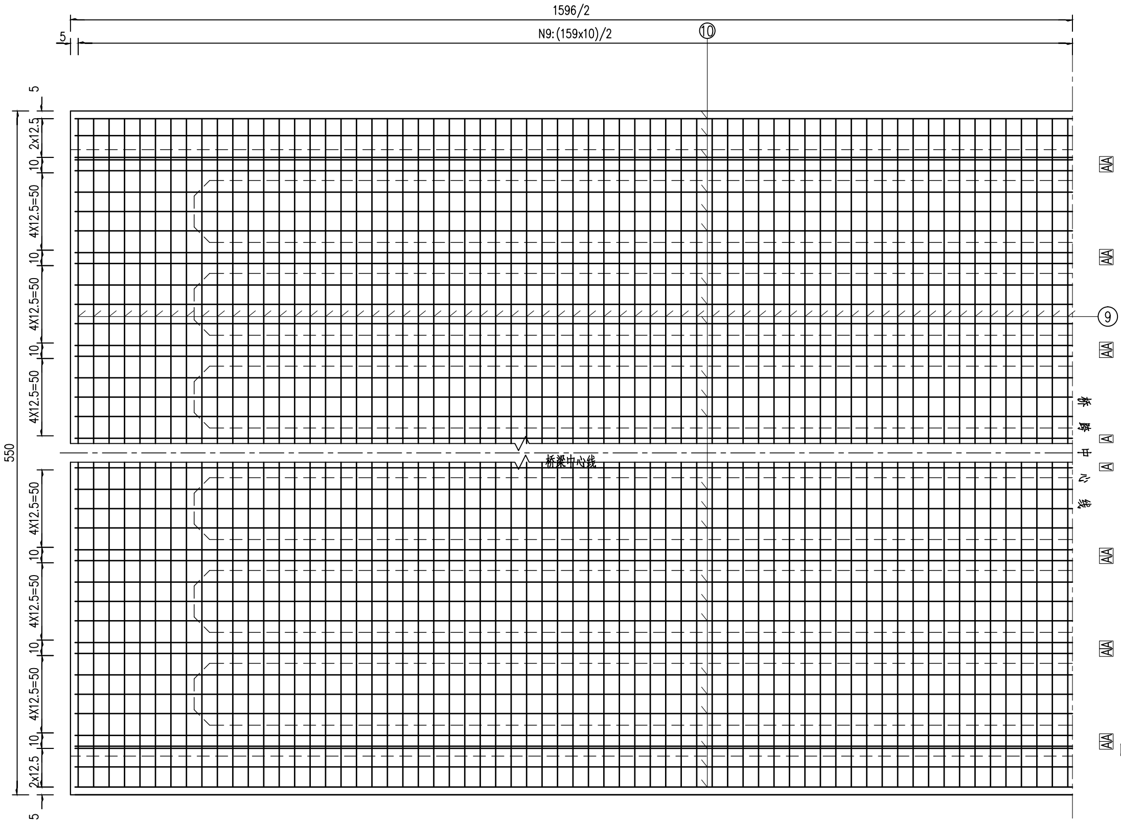
顶板钢筋平面图 1:25
