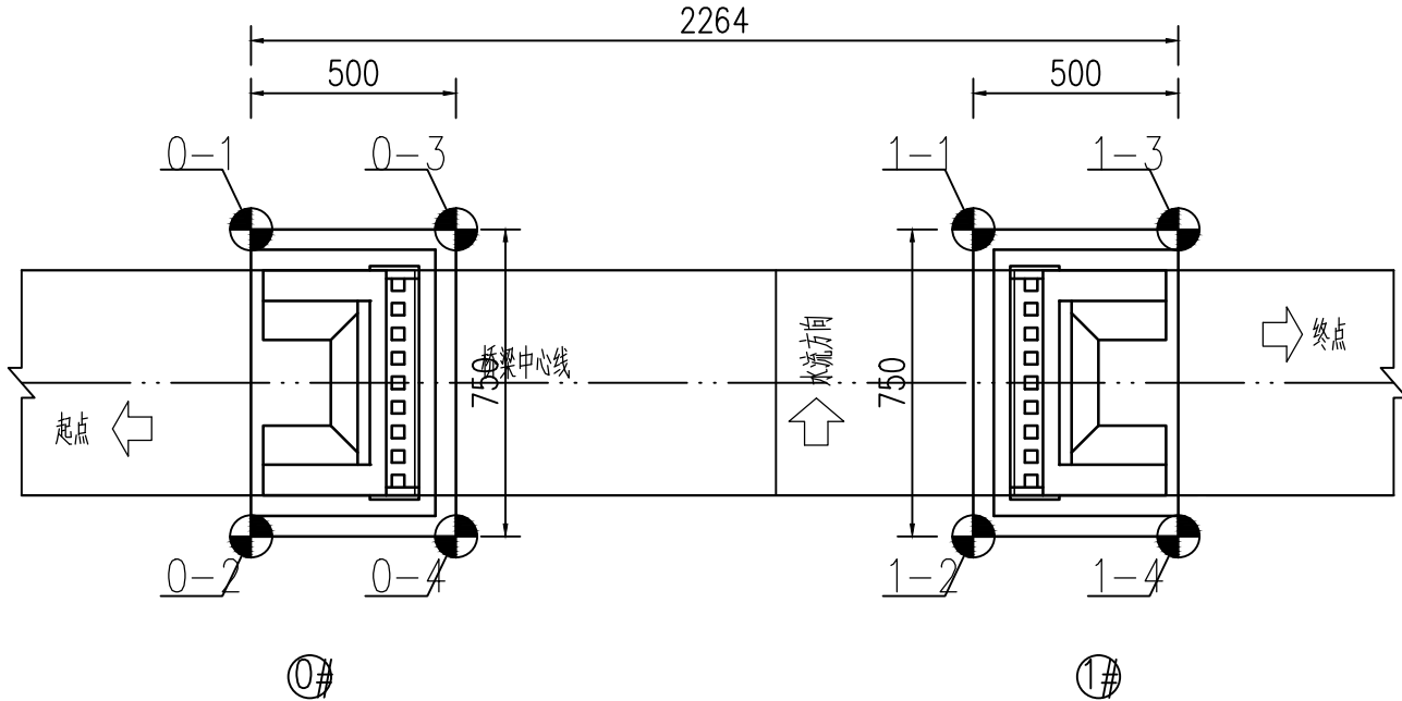
施工坐标放样图 (1:200)
