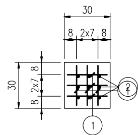
支座垫石钢筋网 1:25
