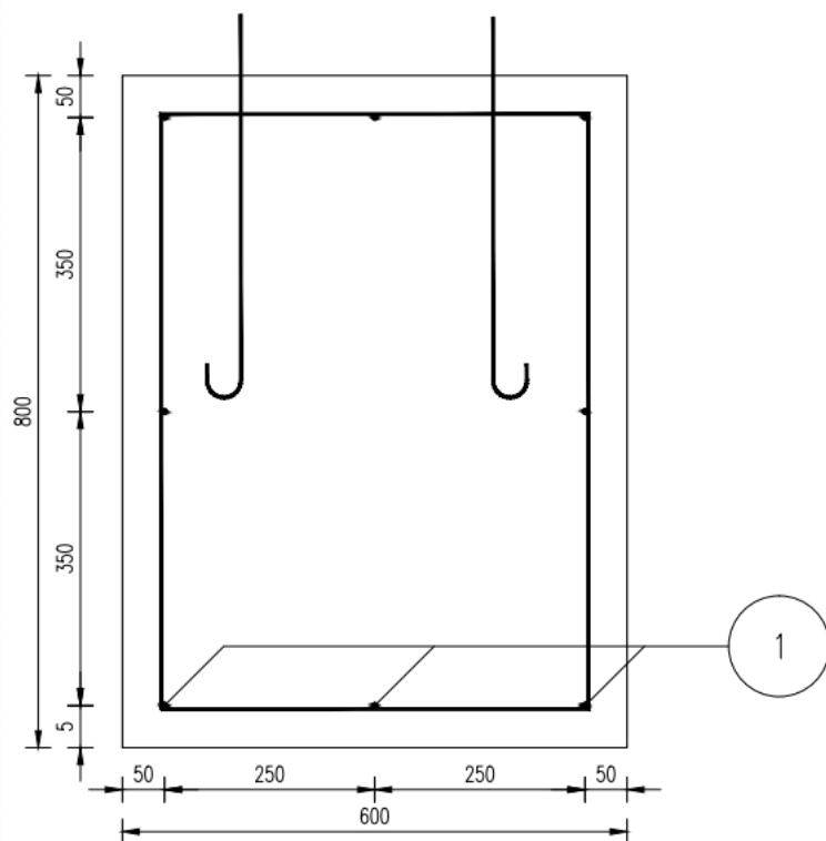
立面图
