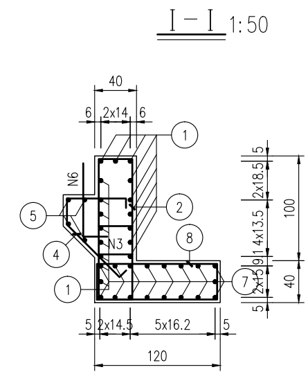
侧墙混凝土横断面 1:50
