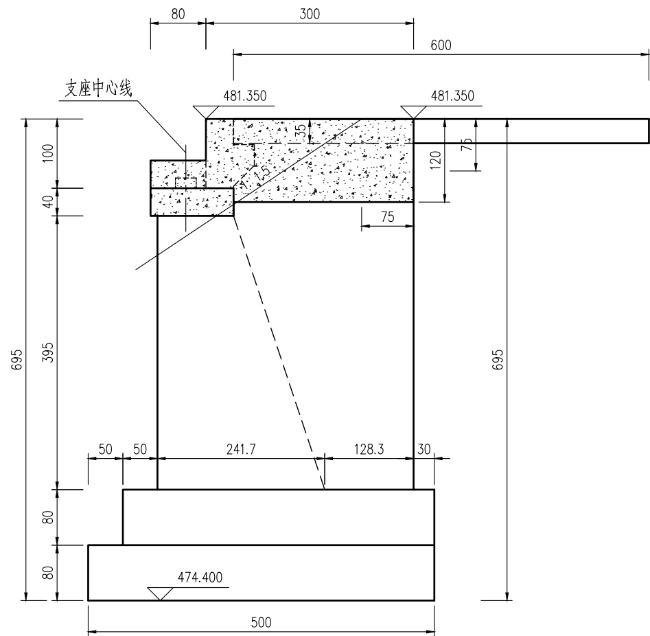
侧面 1:75
