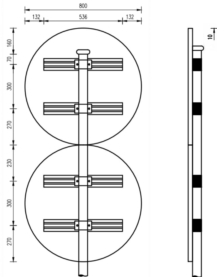
标志板与立柱连接图
