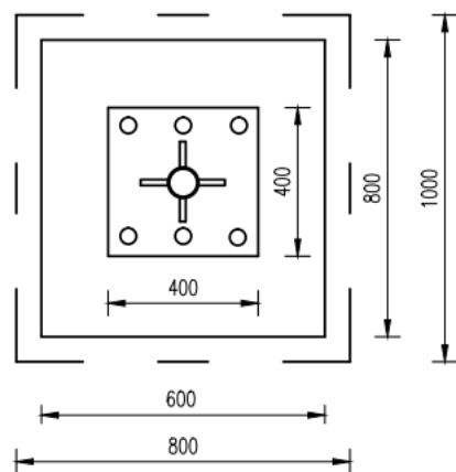
A-A剖面图
