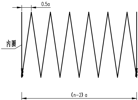
钢筋圈
