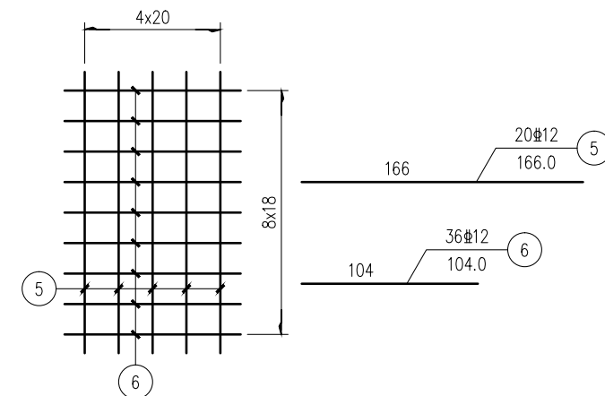
角隅加强钢筋网 1:40
