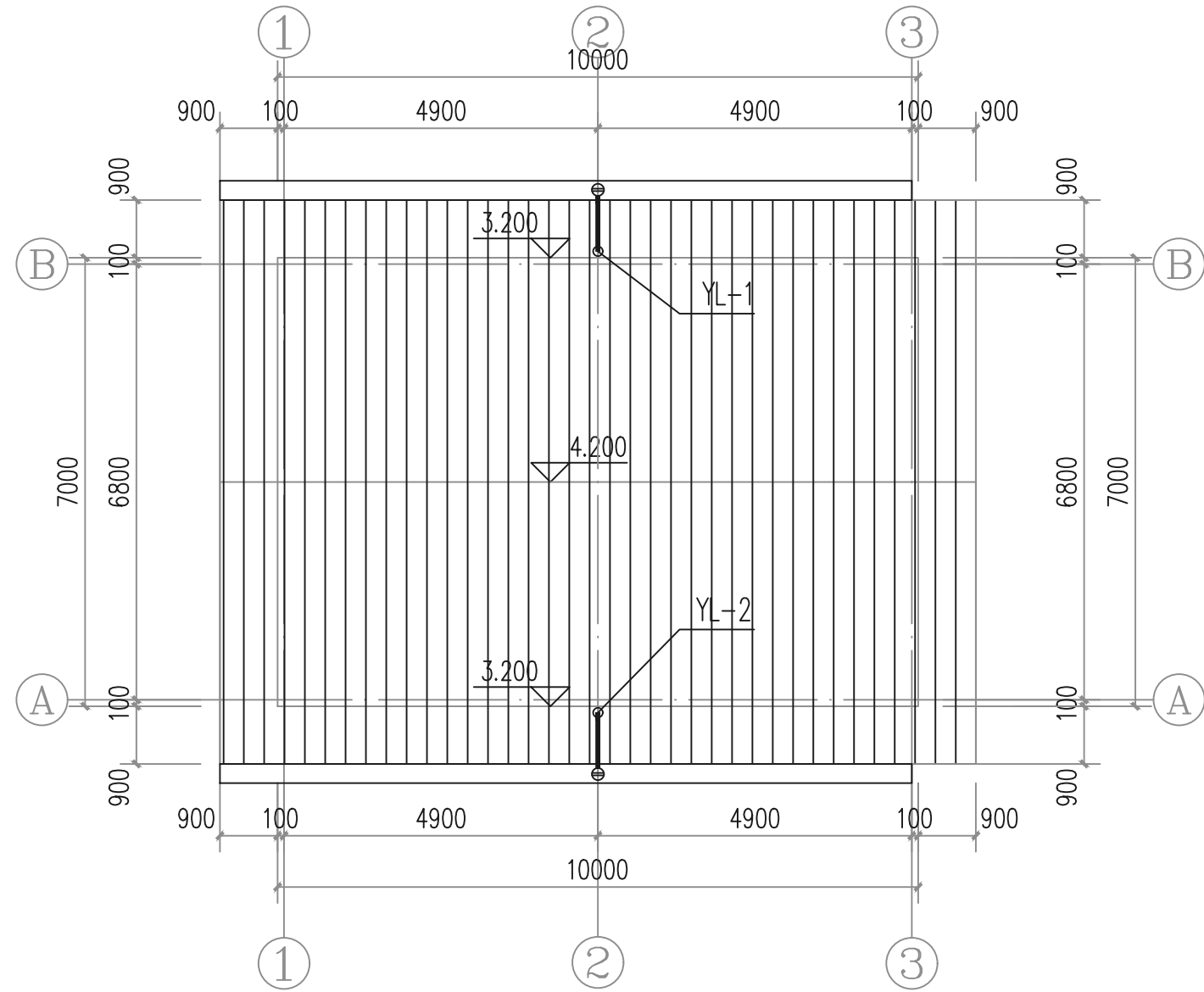
粪房屋顶层给排水平面图 1:100
