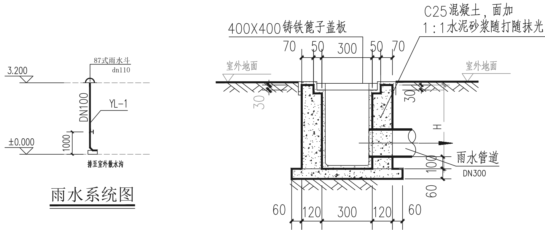
沉沙出水口大样 1:20
