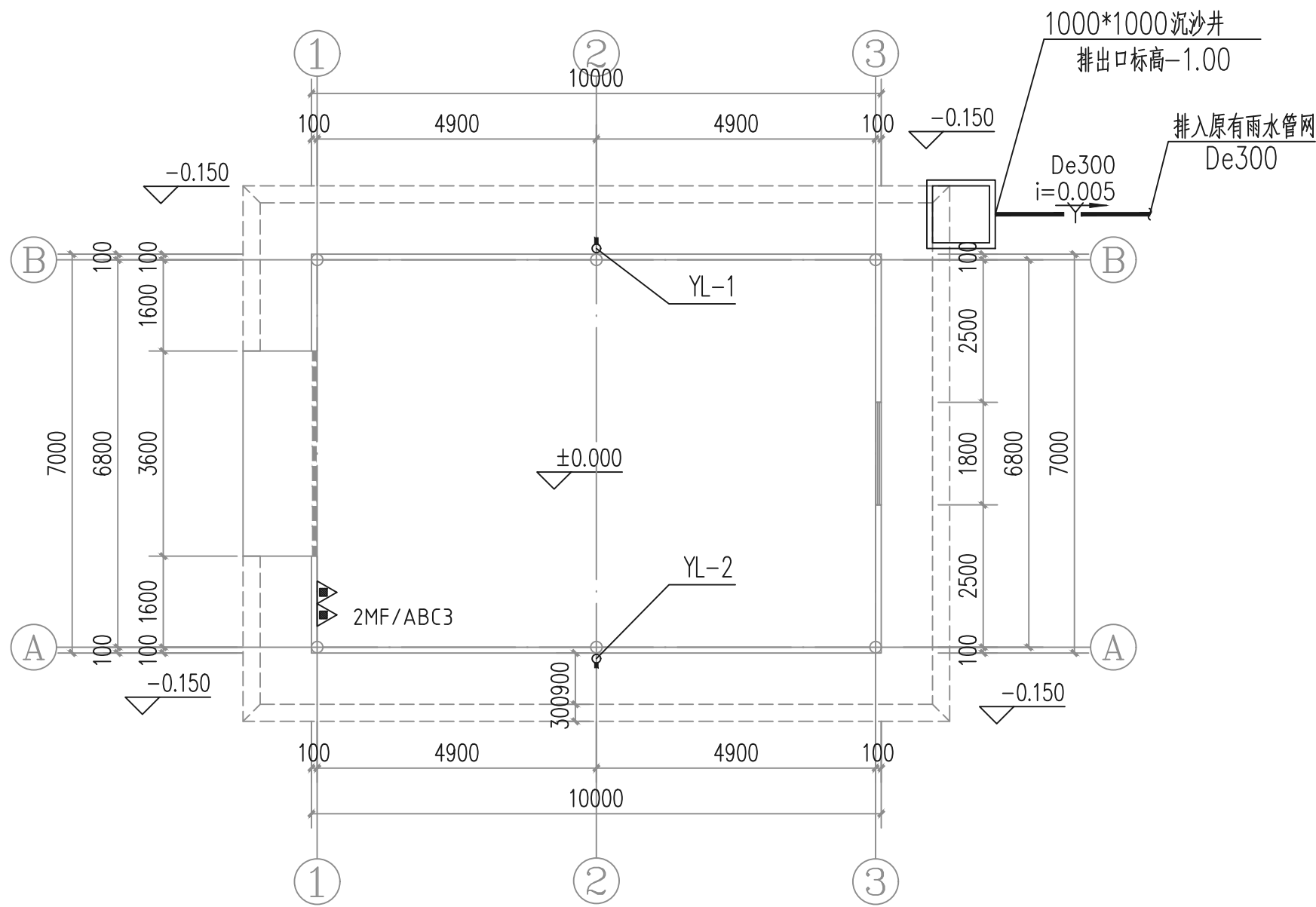
粪房一层给排水平面图 1:100
