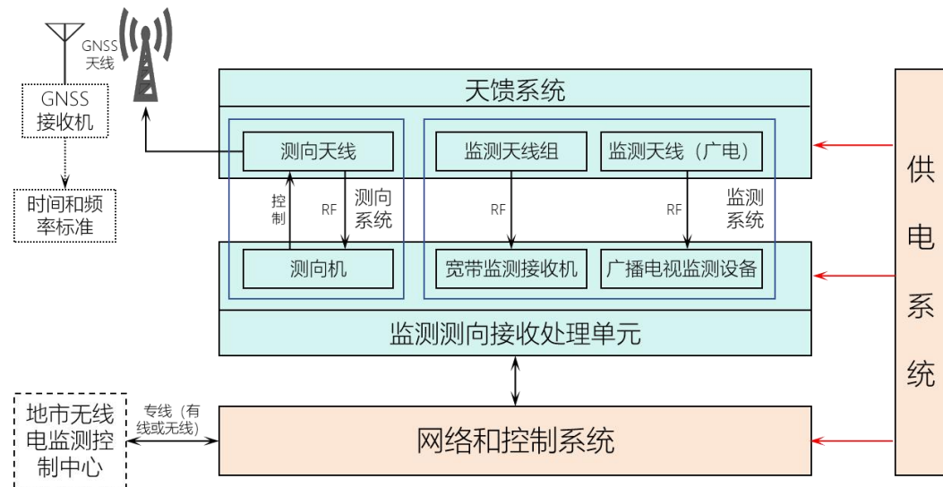
图 2-1 二类可搬移监测站建设架构示意图
