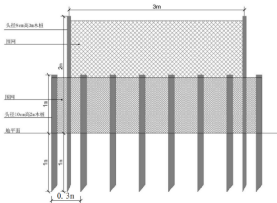
图 4.1-2 围栏网示意图
