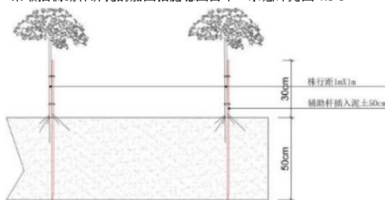
图 4.1-1 辅助杆示意图
