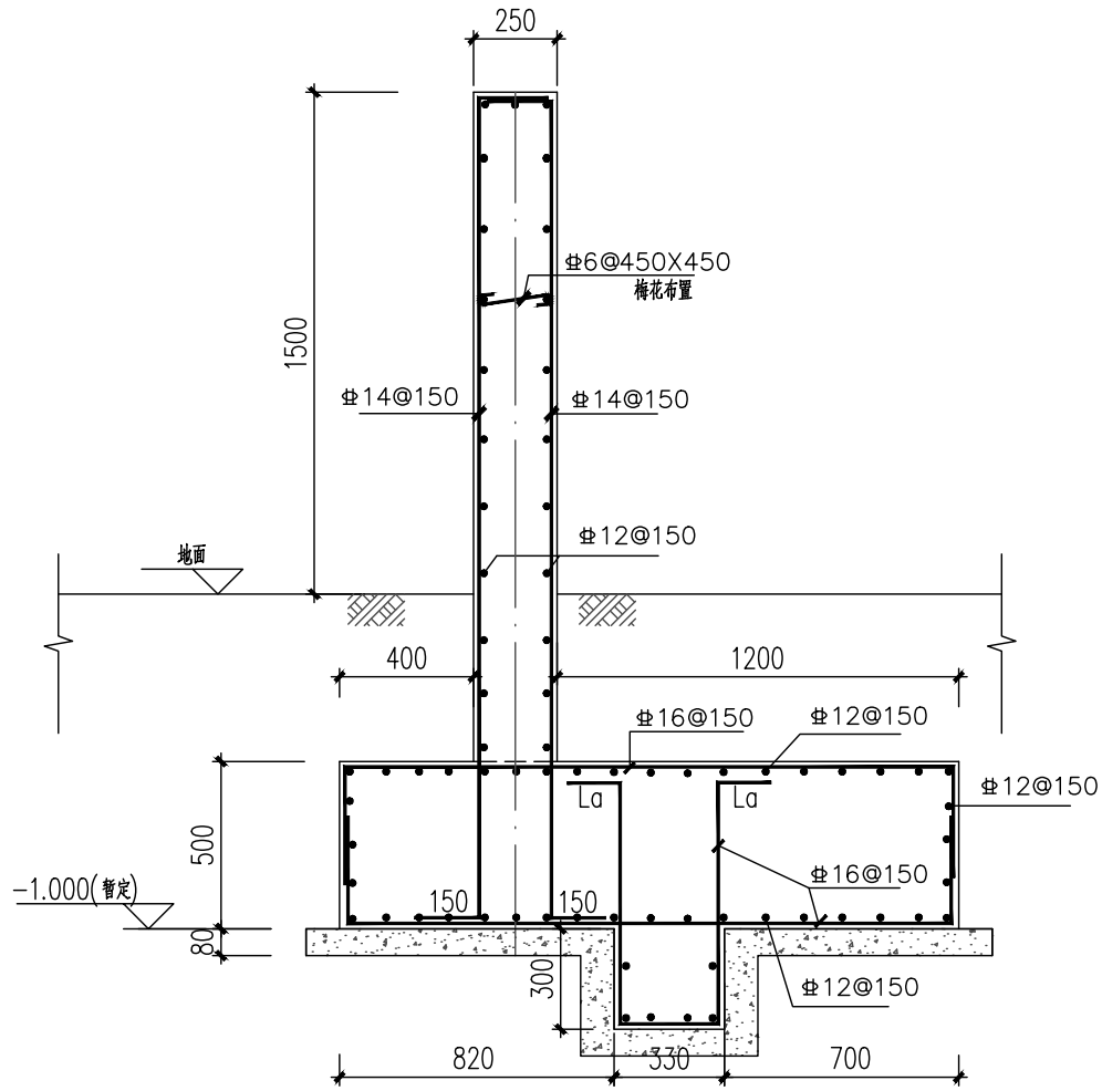
混凝土反边
