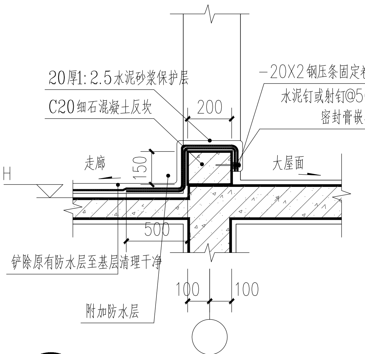
② 反坎防水做法 1:20
