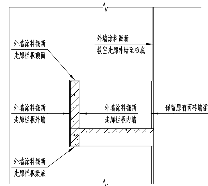
走廊涂料翻新范围示意图 1:150
