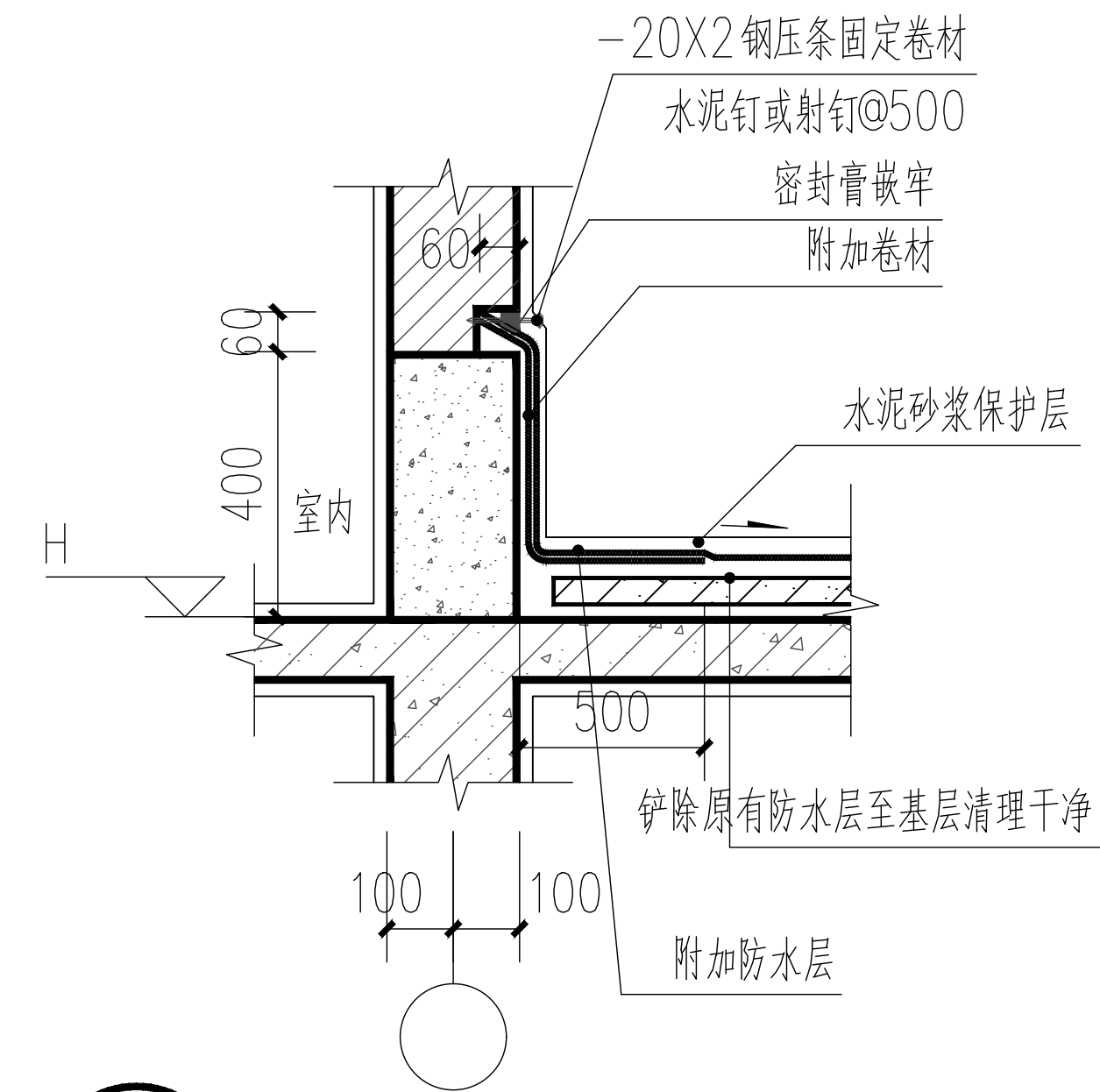
1 砖墙身泛水封口 1:20
