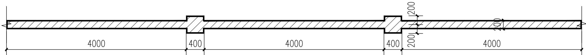
围墙平面图 1:50
