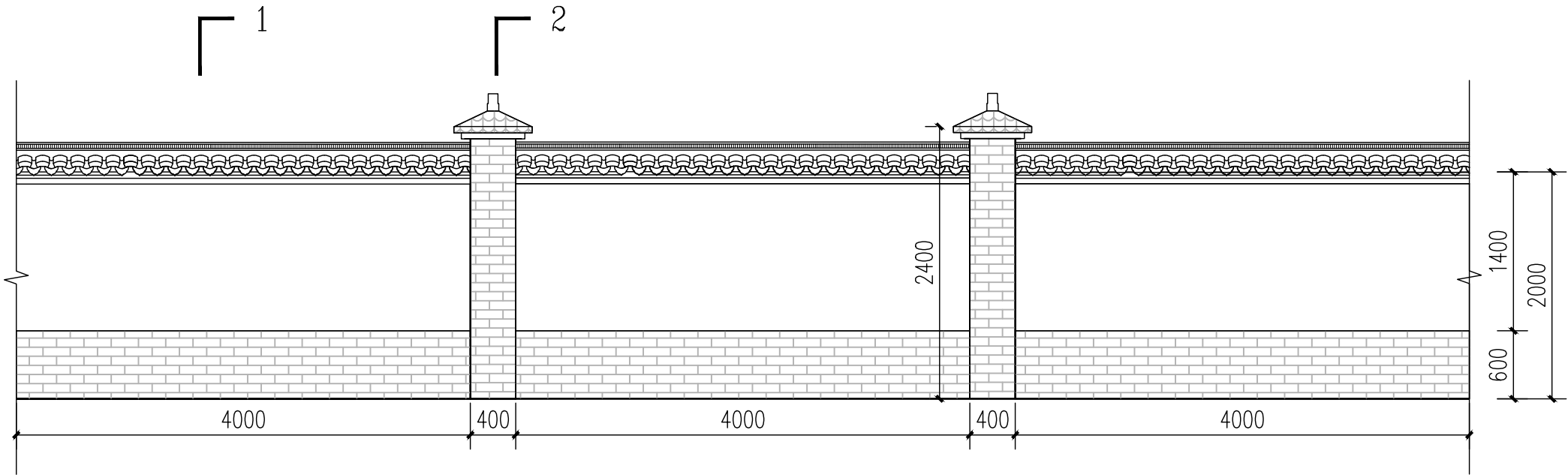
围墙立面图 1:50
