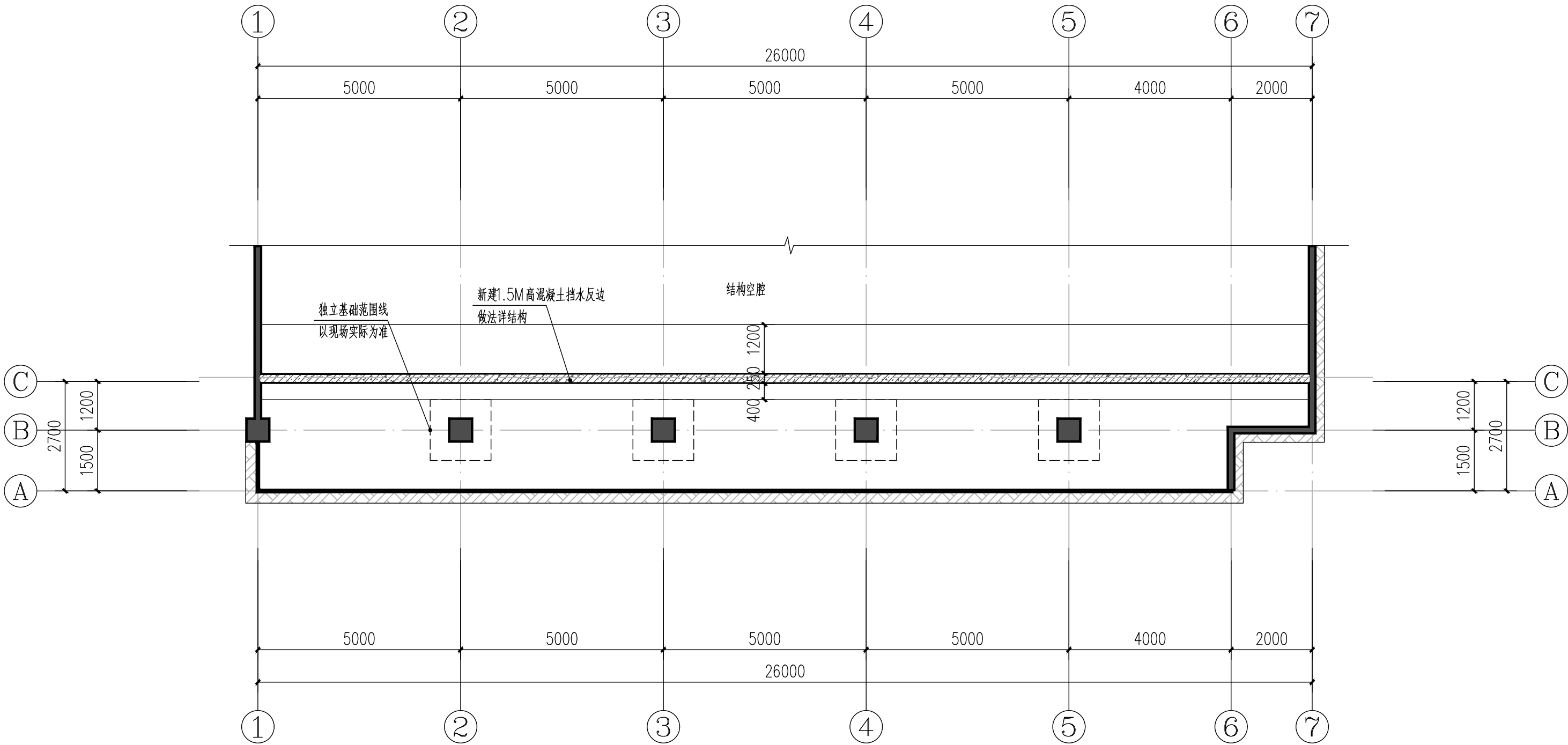
混凝土反边平面图 1:100
