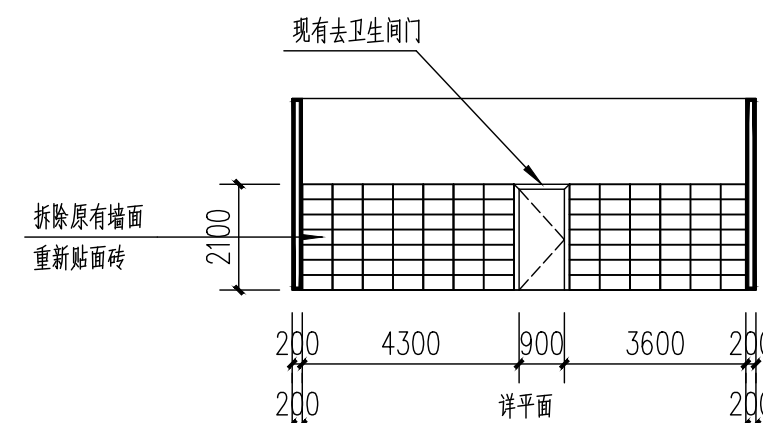
教室靠卫生间处内墙面立面示意图 1:150
