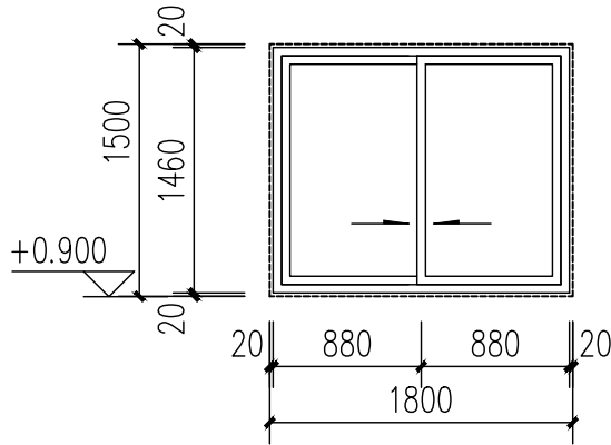
深灰色1.8厚90系列普通铝合金窗+6厚透明钢化白玻璃, 3轨道带金刚纱窗
