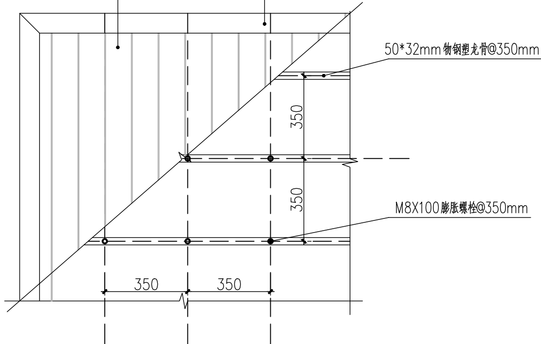
矿物钢塑地板做法大样 1:20
