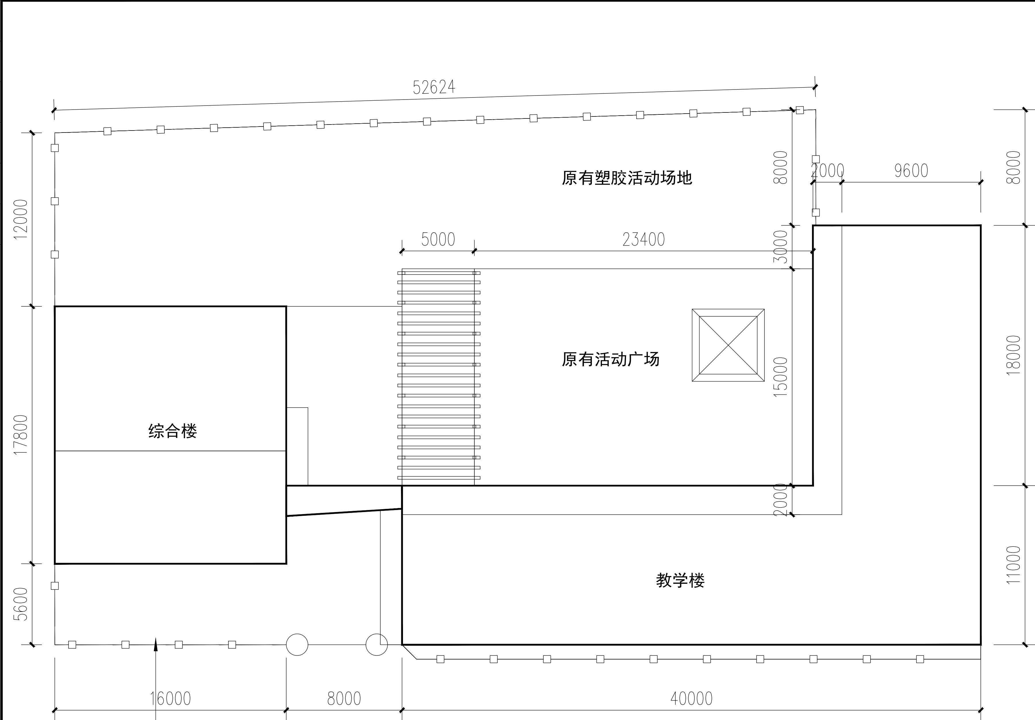
原始总平面示意图 1:300
