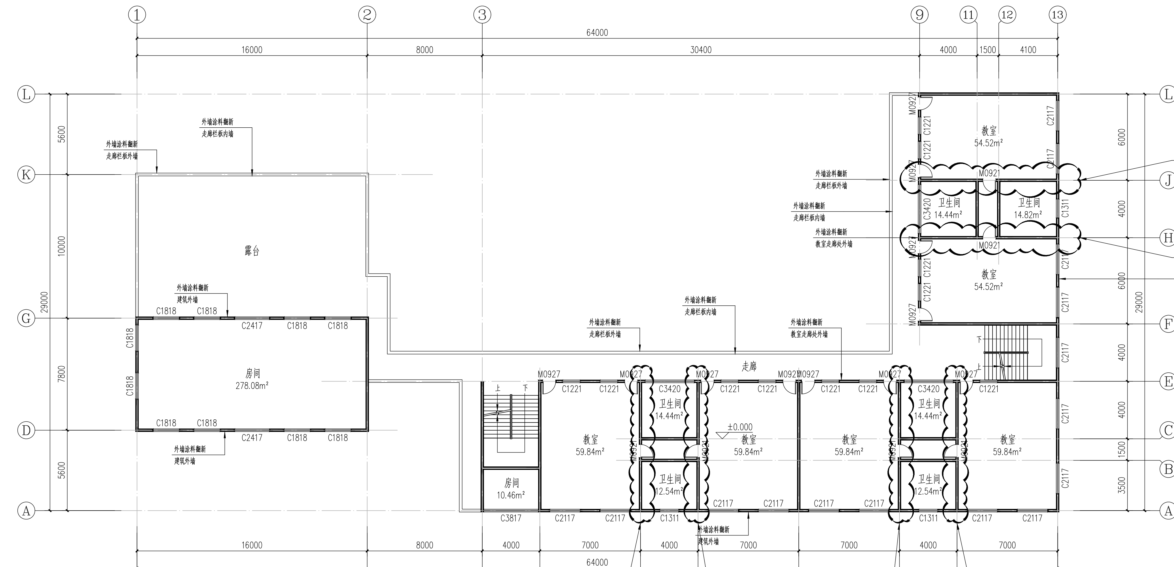
三层平面图 1:150
