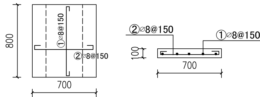
人行桥配筋图
