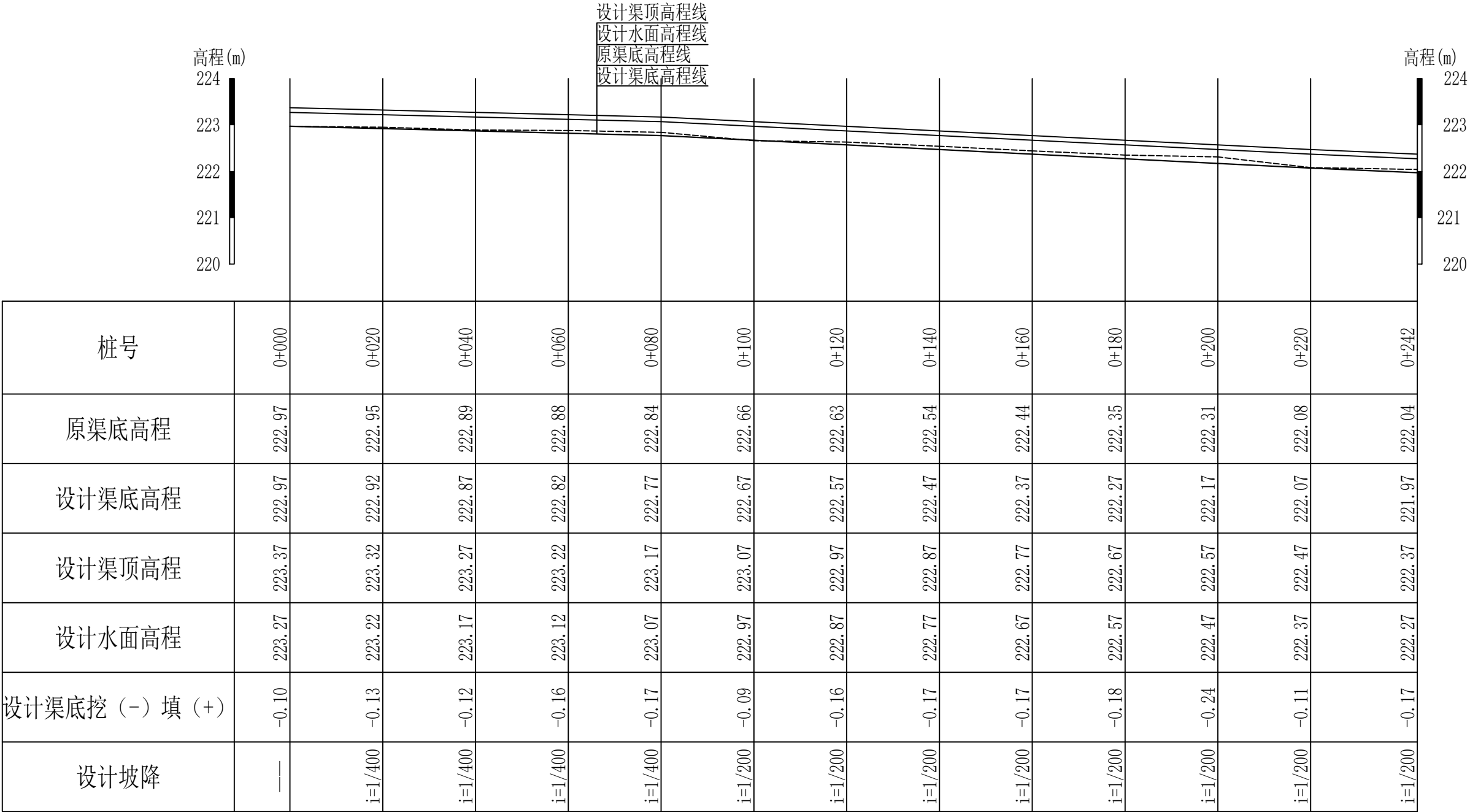
13纵断面
