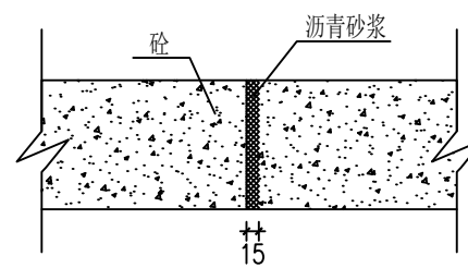
伸缩缝大样图 1: 10
