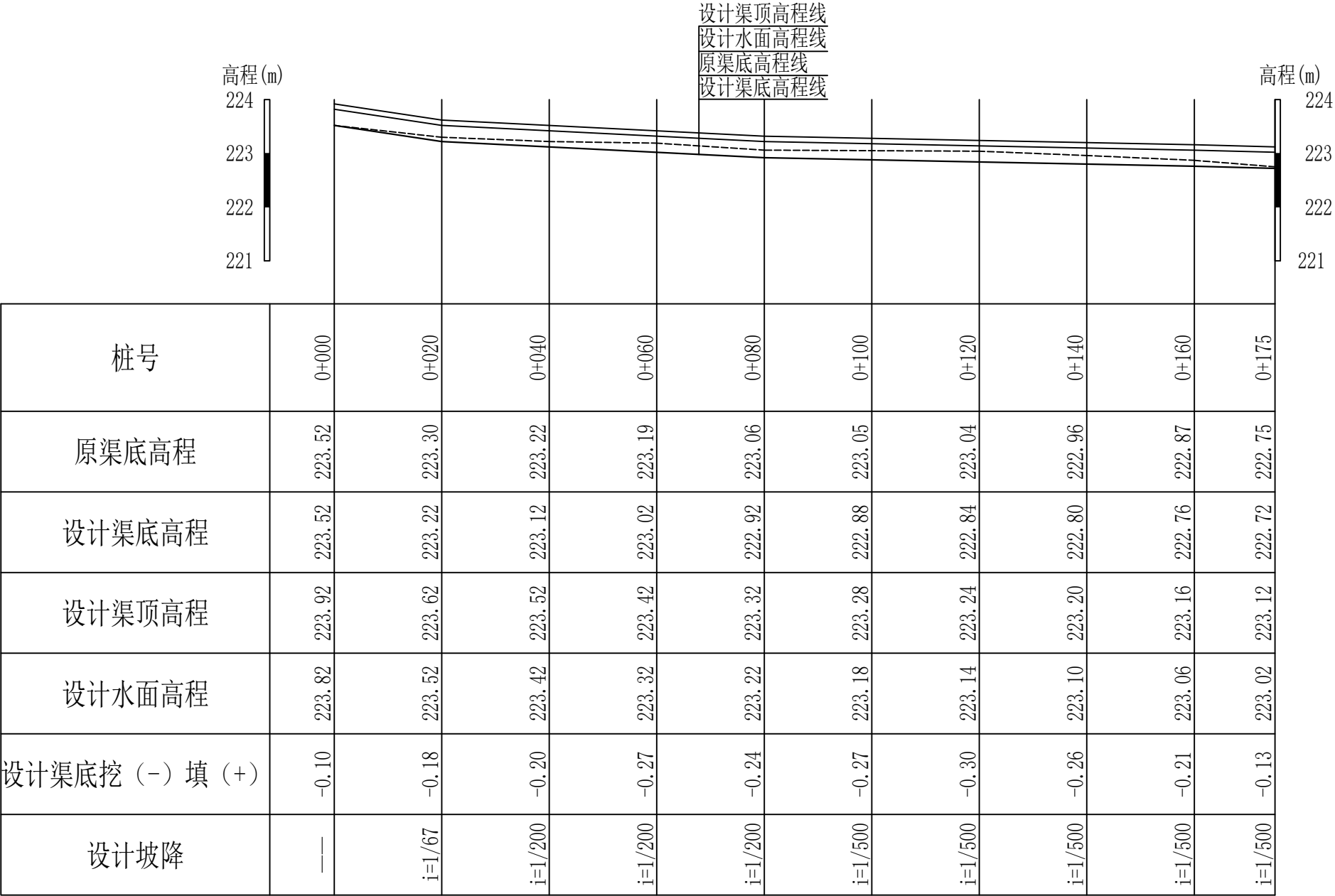
15纵断面 纵向 1:100 横向 1:1000
