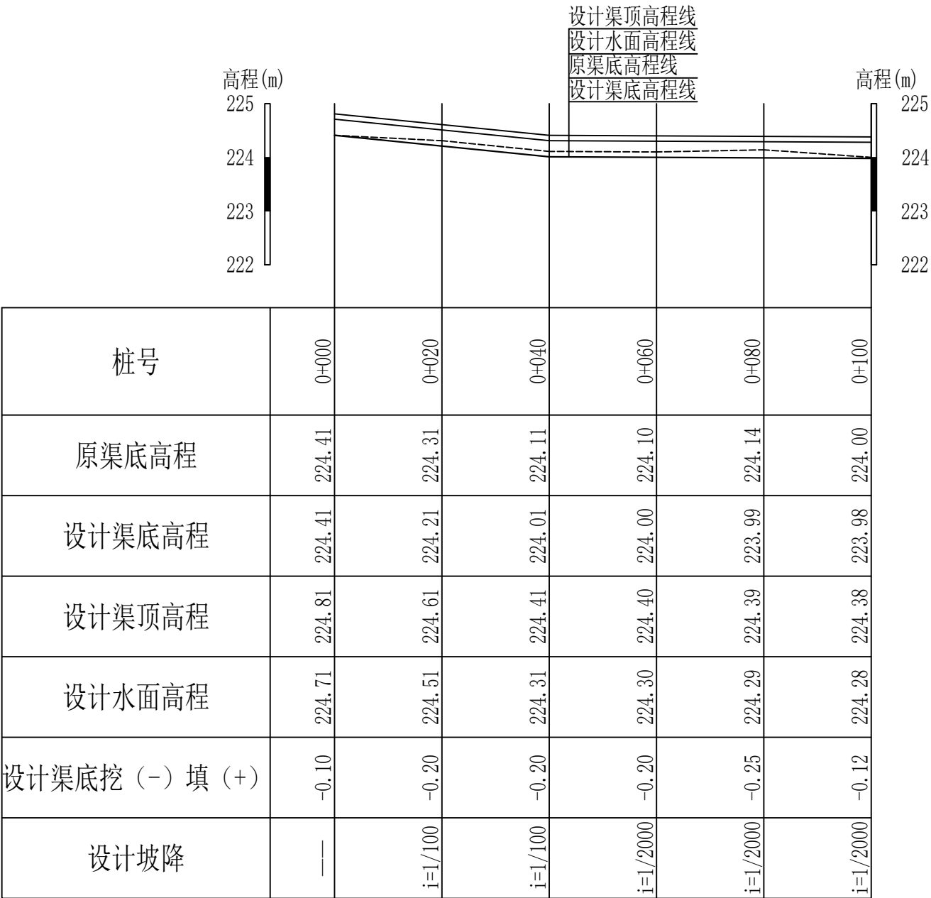
9纵断面 纵向 1:100 横向 1:1000
