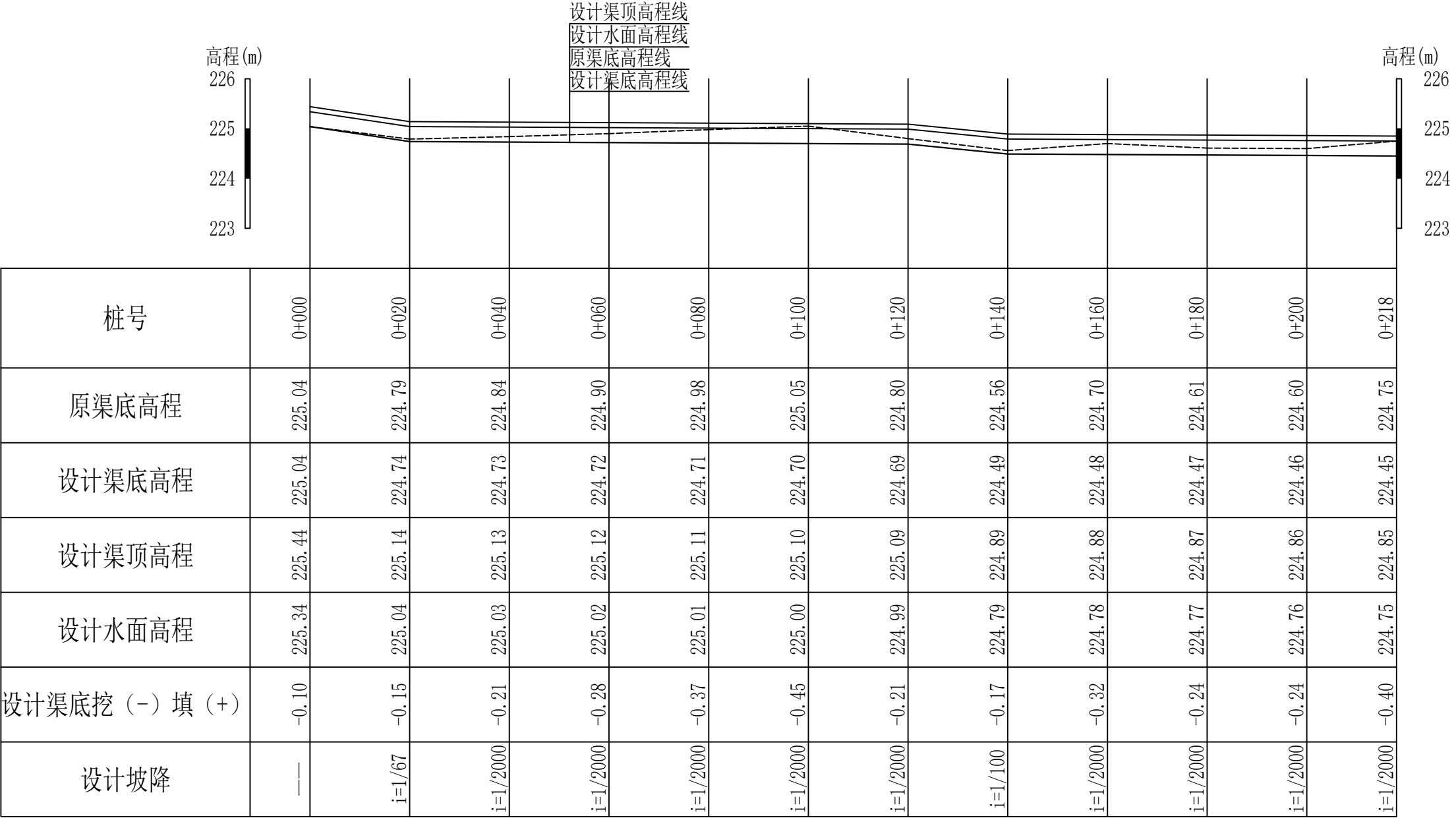
6纵断面 纵向 1:100 横向 1:1000
