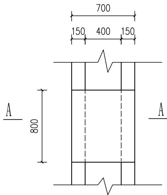
人行桥平面图
