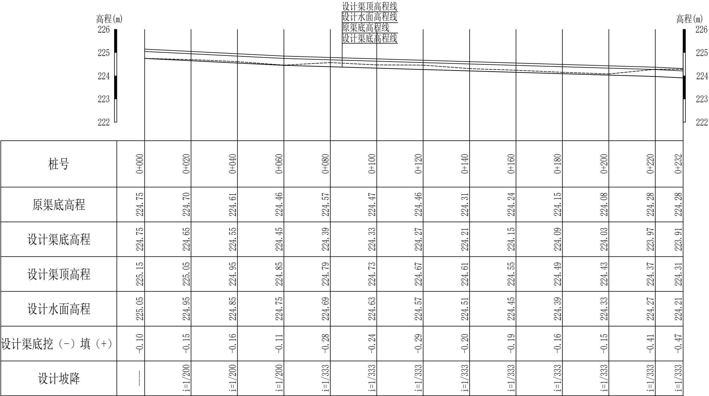
3纵断面 纵向 1:100 横向 1:1000
