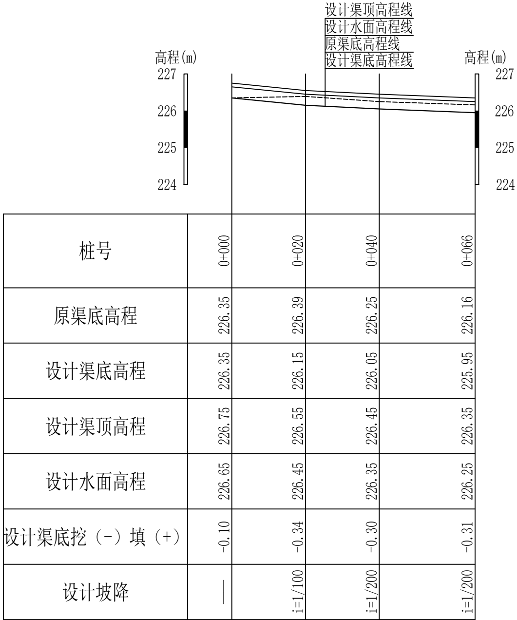
12纵断面 纵向 1:100 横向 1:1000
