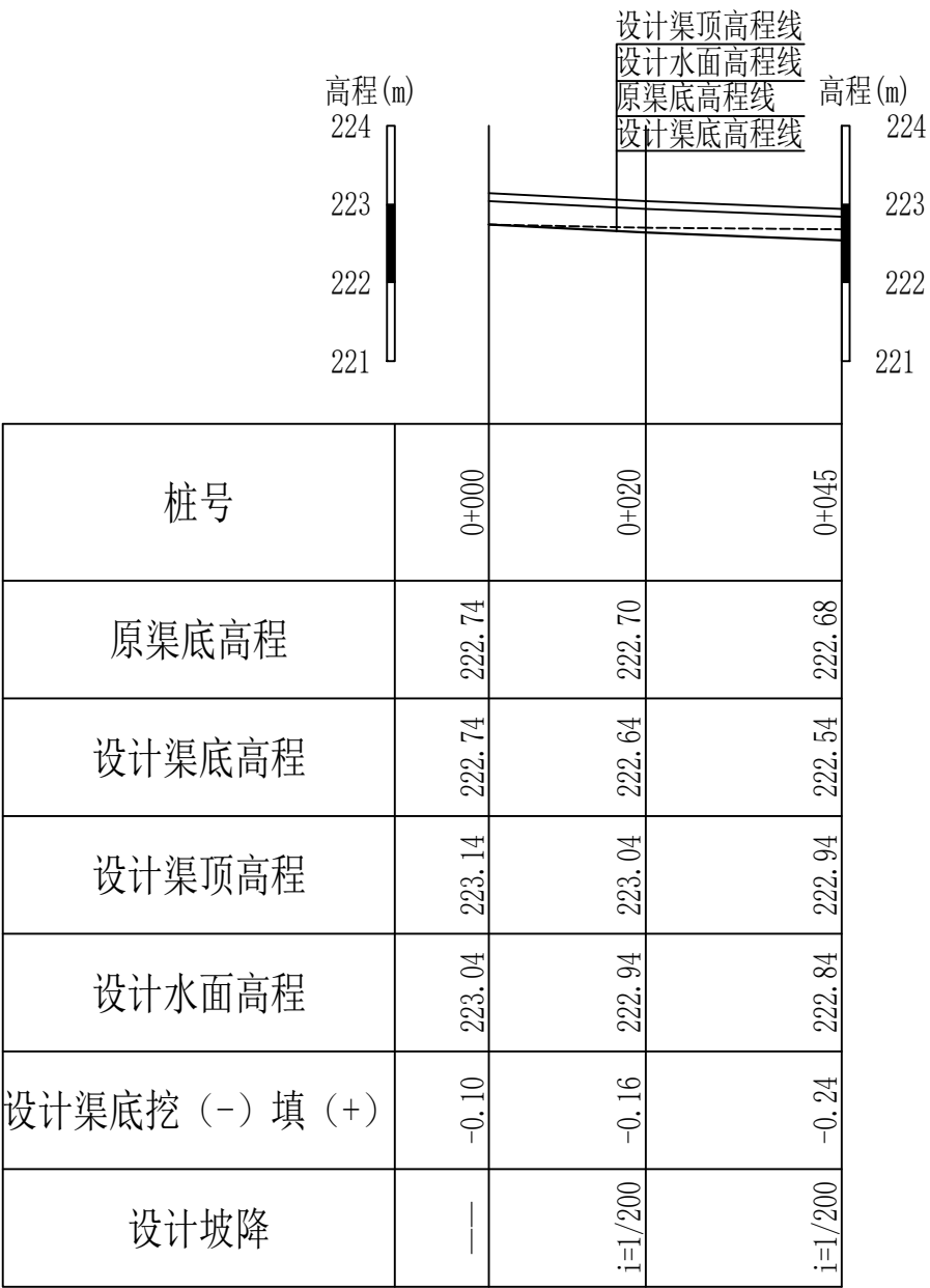
14纵断面 纵向 1:100 横向 1:1000
