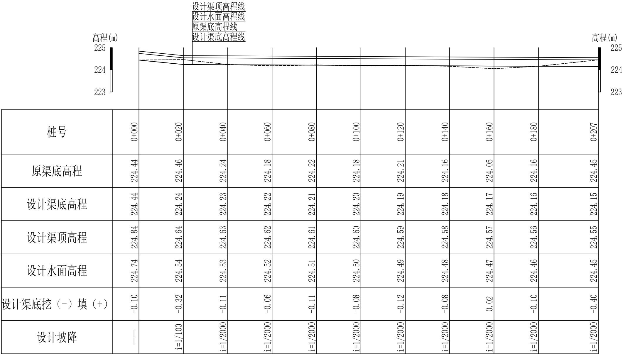
2纵断面 纵向 1:100 横向 1:1000
