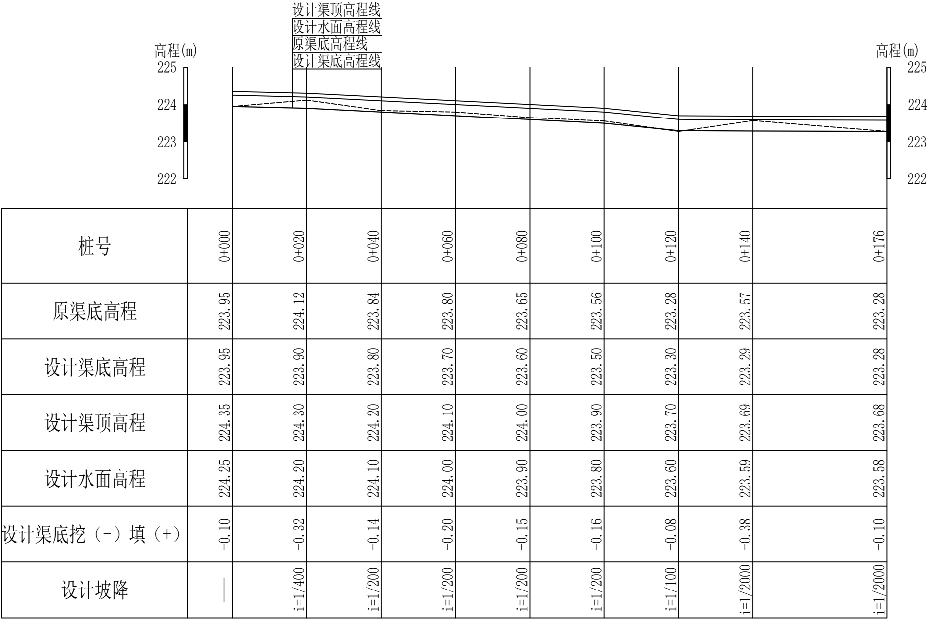
17纵断面 纵向 1:100 横向 1:1000
