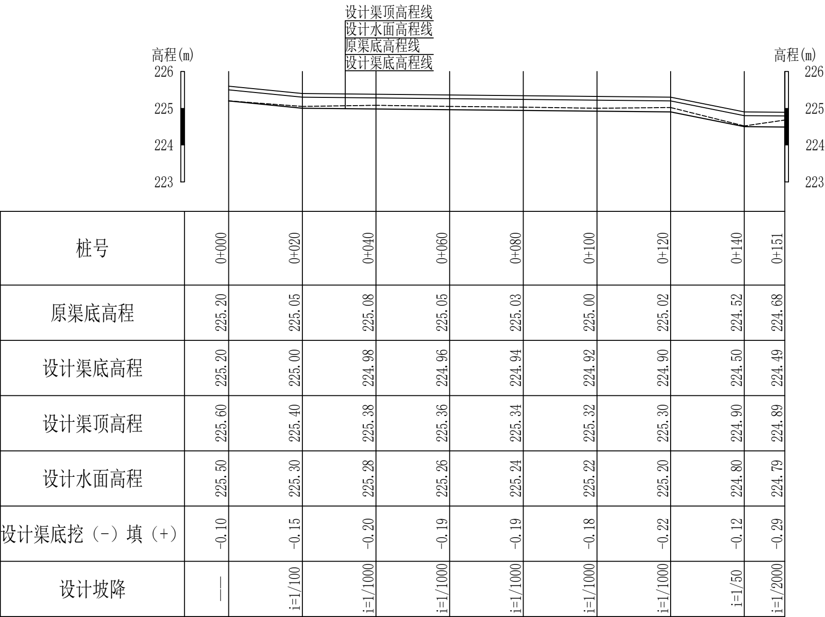
5纵断面 纵向 1:100 横向 1:1000
