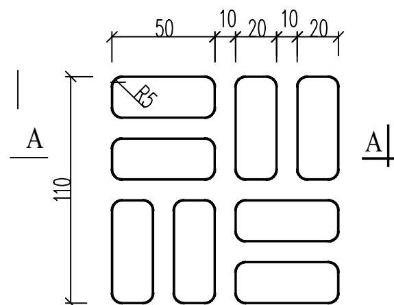
花纹大样
