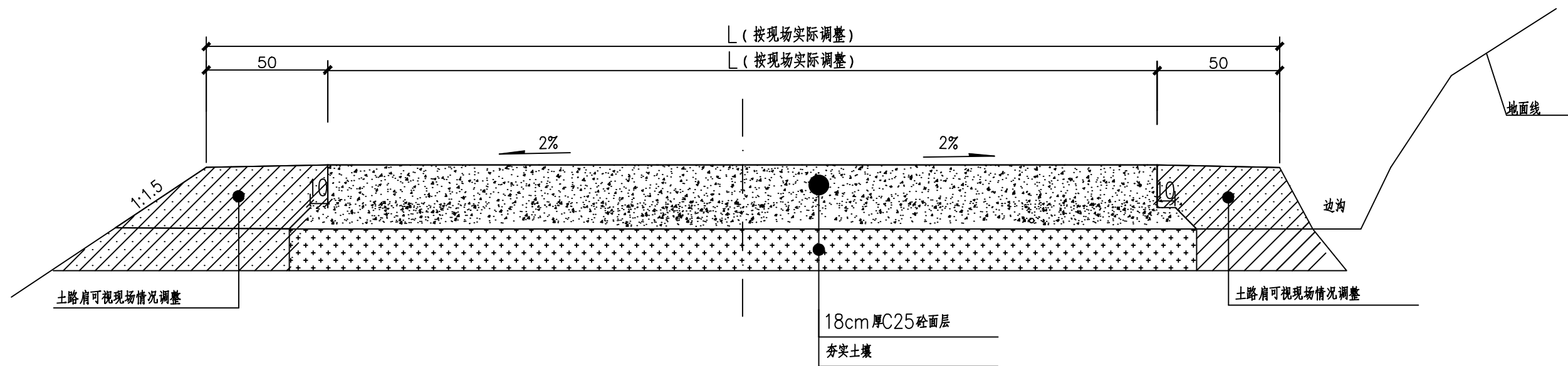
路面结构设计图
