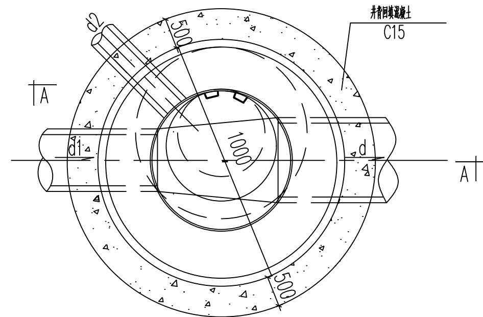
圆形井平面图
