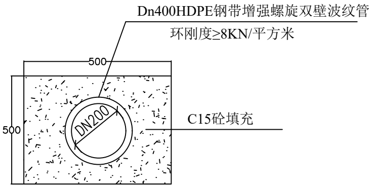
DN200塑料管道管沟槽开挖及回填断面图
