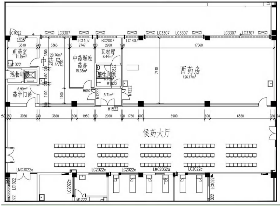
附件 1：中药房及西药房平面图
